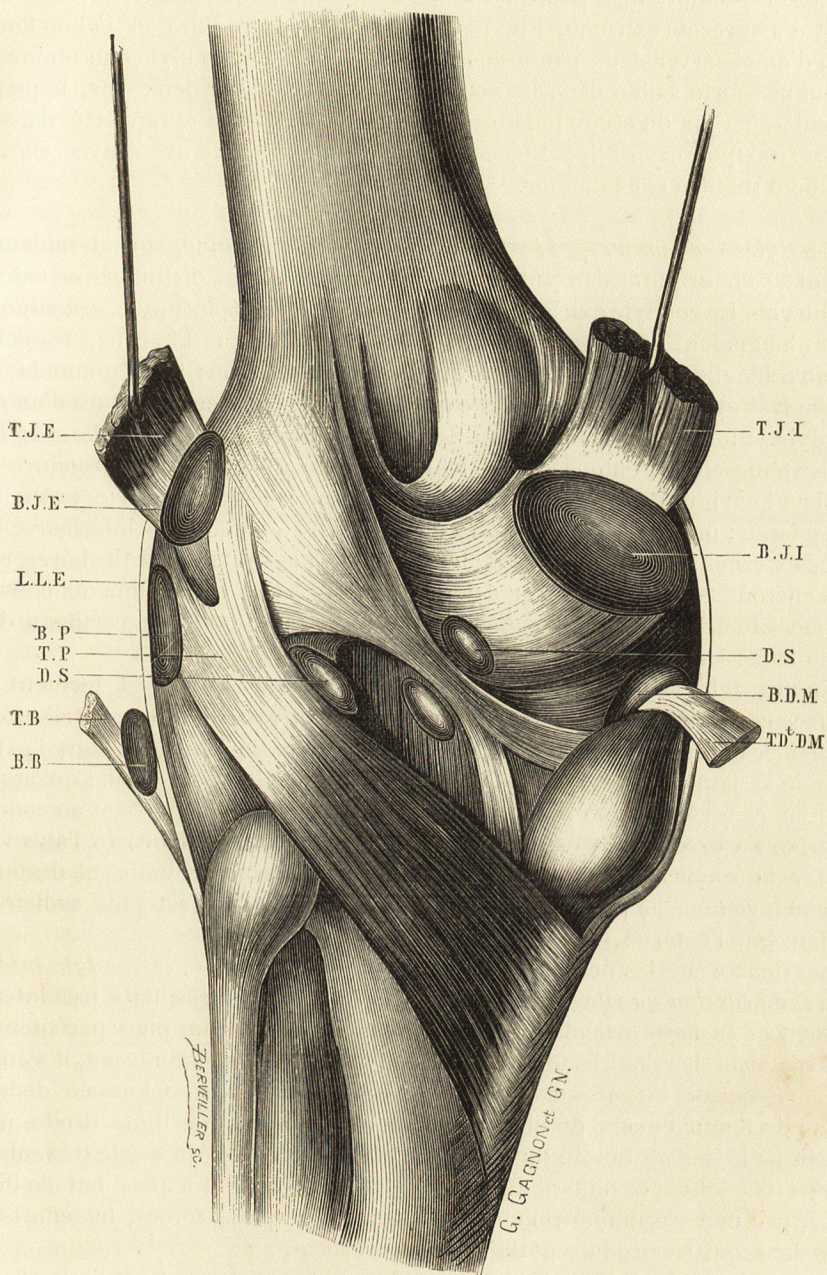
Fig. 296. — Schéma représentant les bourses séreuses du creux poplité.
