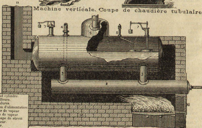
Générateur, ou chaudière à bouilleurs.
