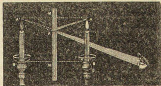
Réflexion de la lumière sur un miroir plan.
