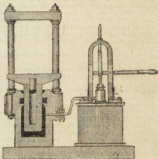
Presse hydraulique.
