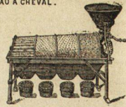
CRIBLE TRIEUR.
