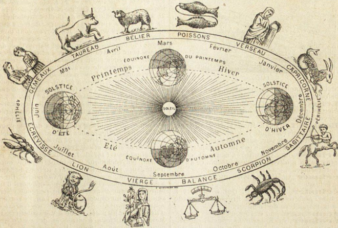
ÉCLIPTIQUE. — Signes du zodiaque.
