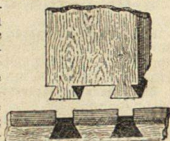
Queue d'aronde.
