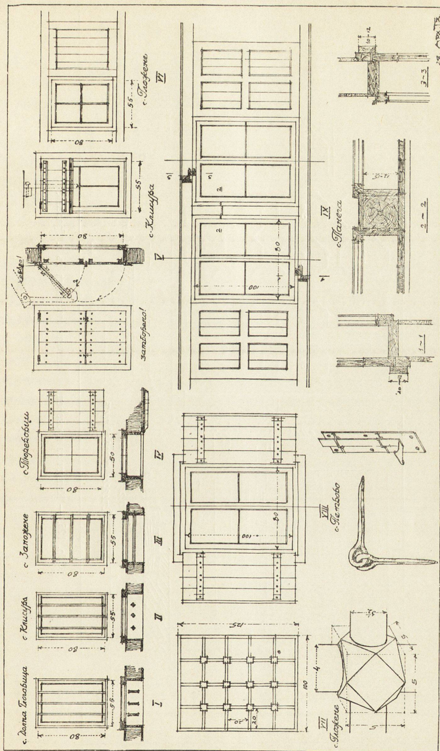
Обр. 124. — Решетки и капаци на прозорци отъ селски кѣши.
