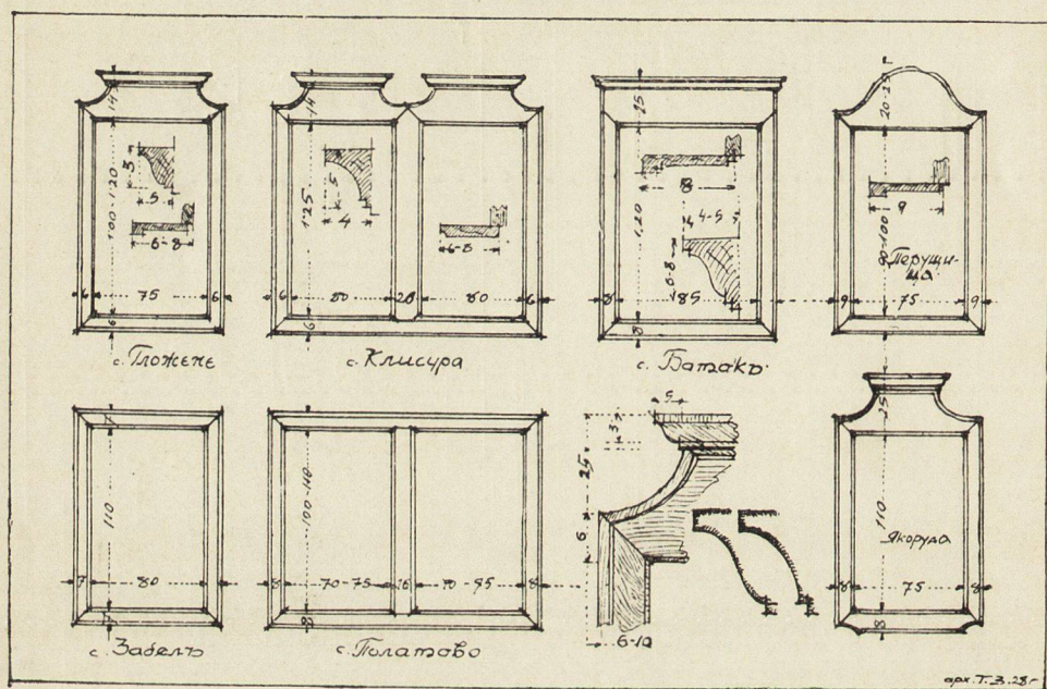
Обр 122. — Дървени рамки на прозорци отъ селски кѣщи.
