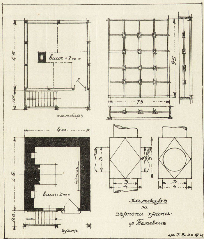
Обр. 116. — Хамбаръ въ гр. Тетевенъ.
