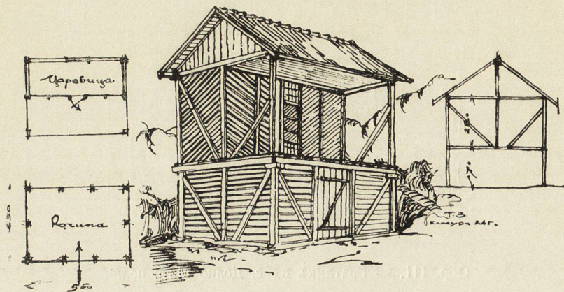
Обр. 113. — Дъсченъ кошъ за царевица.
