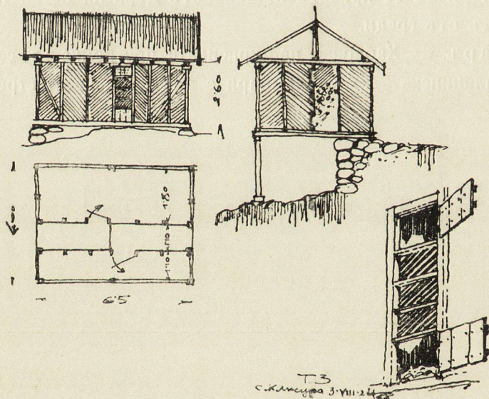
Обр. 114. — Дъсченъ кошъ за царевица.
