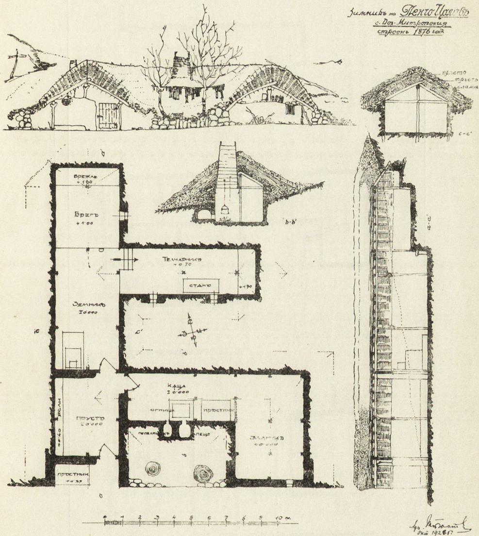
Обр. 97. — Троглодитна кжща въ с. Долна-Митрополия — плѣвенско.
