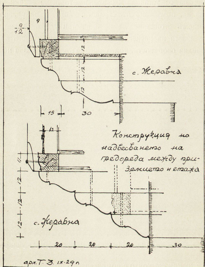
Обр. 43. — Детайл отъ жеравненска кжща.
