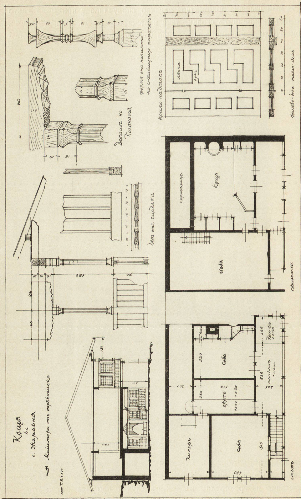
Обр. 35. — Къща въ с. Жеравна разпредѣление.
