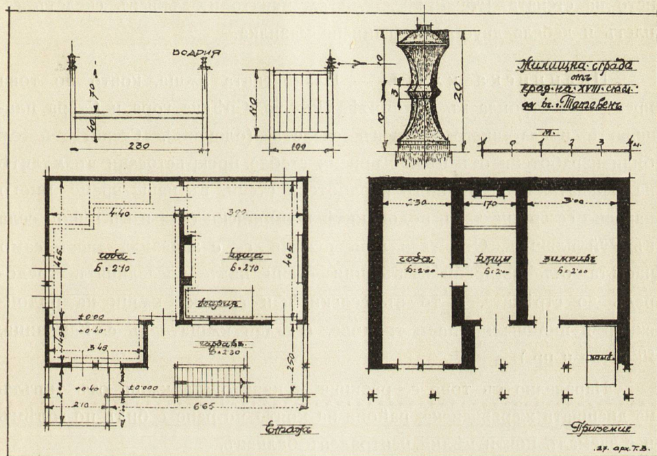
Обр. 14. — Кжща отъ края на XVIII вѣкъ въ гр. Тетевенъ. Планъ.
