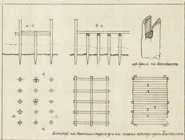
Обр. 9. — Конструкция на долния строежъ на наколнитъ постройки въ Кастиионе.
