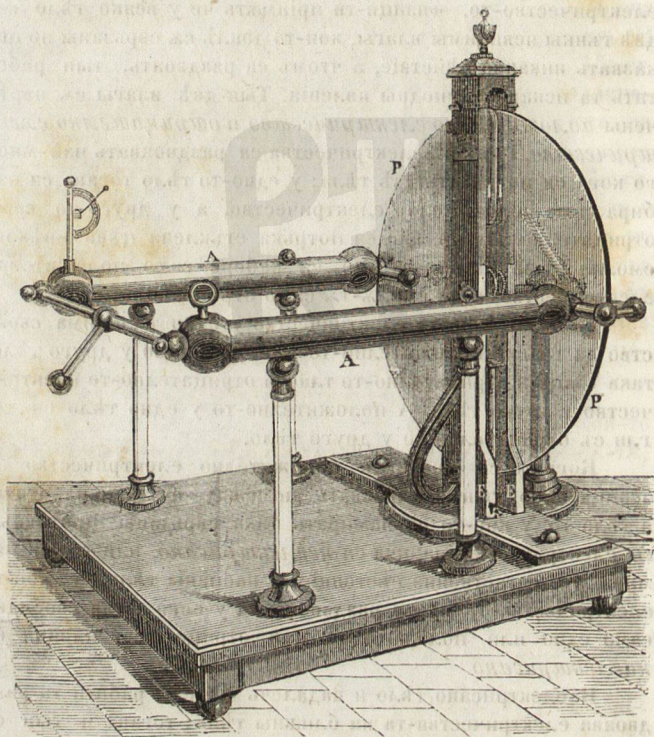
Фиг. 5. Електрическа машина.
