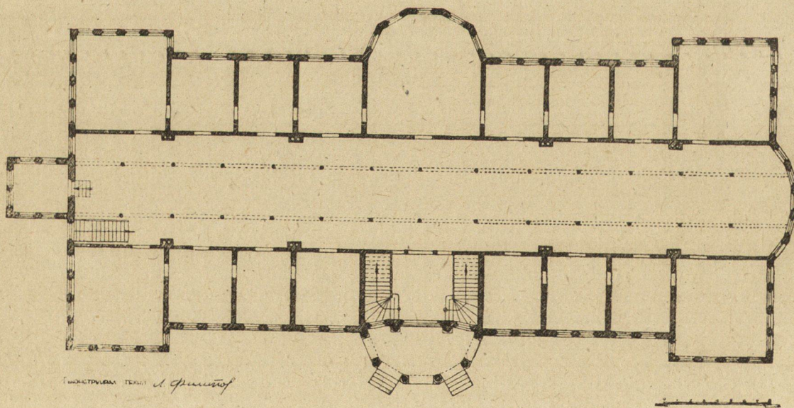
76. Търново. Бившият турски конак (1872—1876) — разпределение на партерния етаж (реконструкция: Леон Филипов, септ. 1951 г.)
