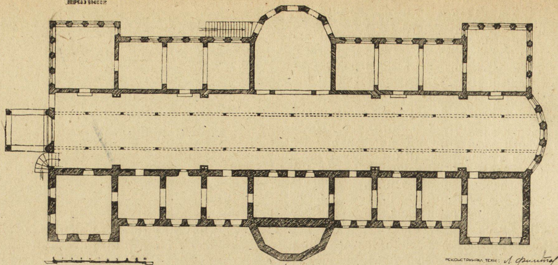
45. Търново. Бившият турски конак (1872—1876) — разпределение на приземието (реконструкция: Леон Филипов — Търново септ. 1951 г.)
