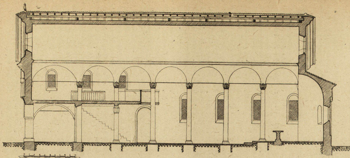
9. Търново. Църквата „Св. Богородица“ (1842—1844), напълно разрушена при земетресението 1913 г.—надлъжен разрез
