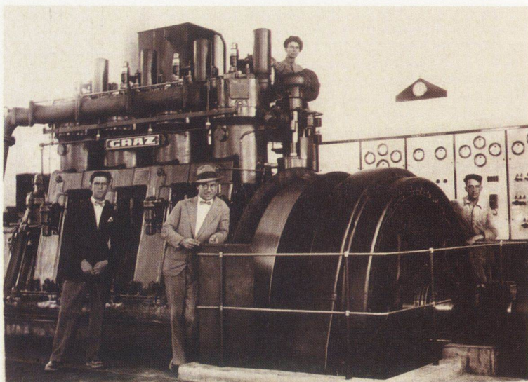
Дизеловият двигател на електроцентралата в Сливен, 20 септември 1928 г.
