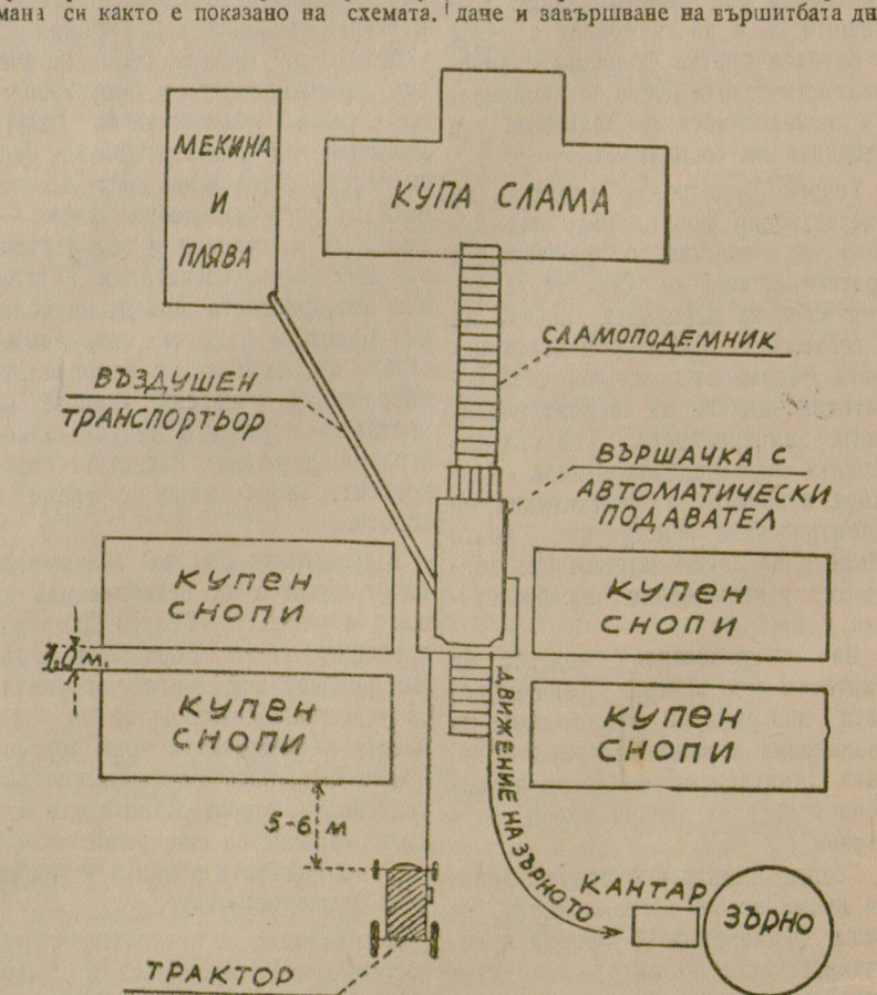
СХЕМА НА ВЪРШАЧНИЯ ХАРМАН, КЪДЕТО Е РАБОТИЛ Н. БРЕДЮК В 1950 ГОД. НА ВЪРШАЧКА МС-А
