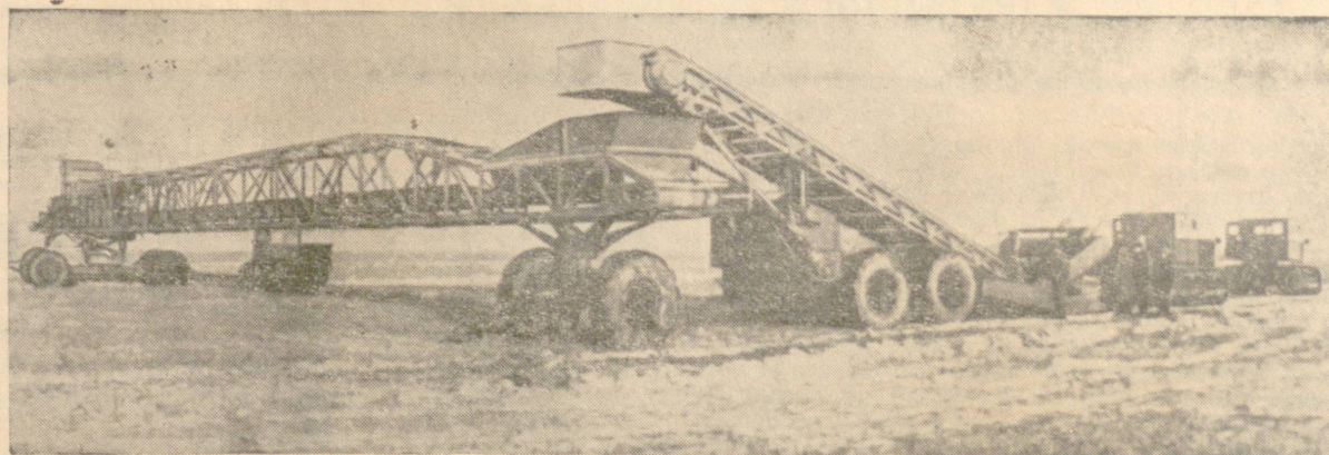
НА СНИМКАТА: Нова мощна машина — землекопен струг „Д — 264“, предназначен за работа в строителството на плавателни и големи магистрални оросителни канали. Изкопаната пръст се изхвърля на повече от 45 метра настрана от мястото на изкопа. Машината се движи с помощта на три трактора „С — 80“. Проектната производителност на машината е 1,500 кубически метра в час.
