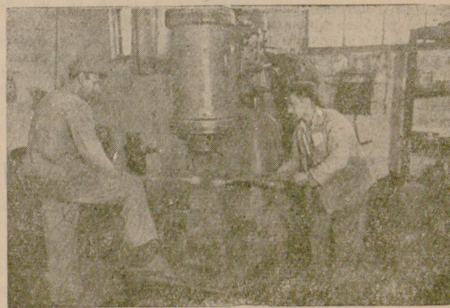
Разнообразни и сложни са детайлите, които се изработват в ковашкия цех на ДМЗ „Червена звезда“ в с. Дебелец, Търново. На снимката: Ковачите Тодор Дончев и Иван Петров работят на автоматичния чук.
