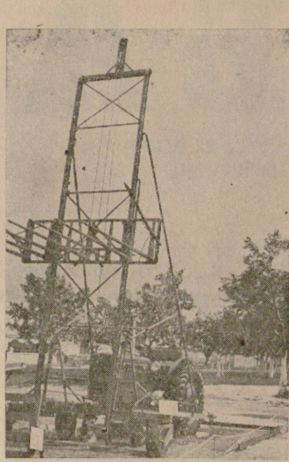
На снимката: Сеносъбирачка „СТУ—07“, която Съветският съюз показа на Пловдивския панаир. Тя има полезен товар 700 кг и височина на издигането 10—22 метра.
