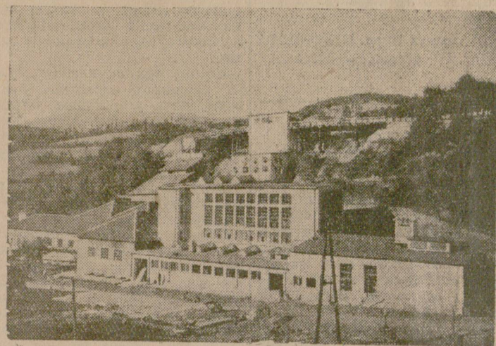
Изглед от новопостроената флотационна фабрика в мина „Чипровци“, Михайловградско.
