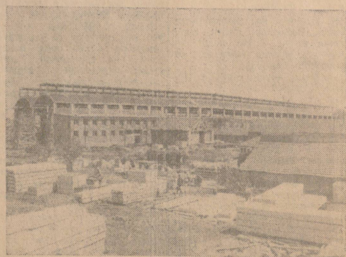
Върху площ от 7,500 квадратни метра се изгражда разширението на каучуковия завод „Г. Димитров“—София. Строителите са обещали да преодат строежа завършен до 1 ноември т. г. На снимката: Общ изглед от строежа на разширението.
