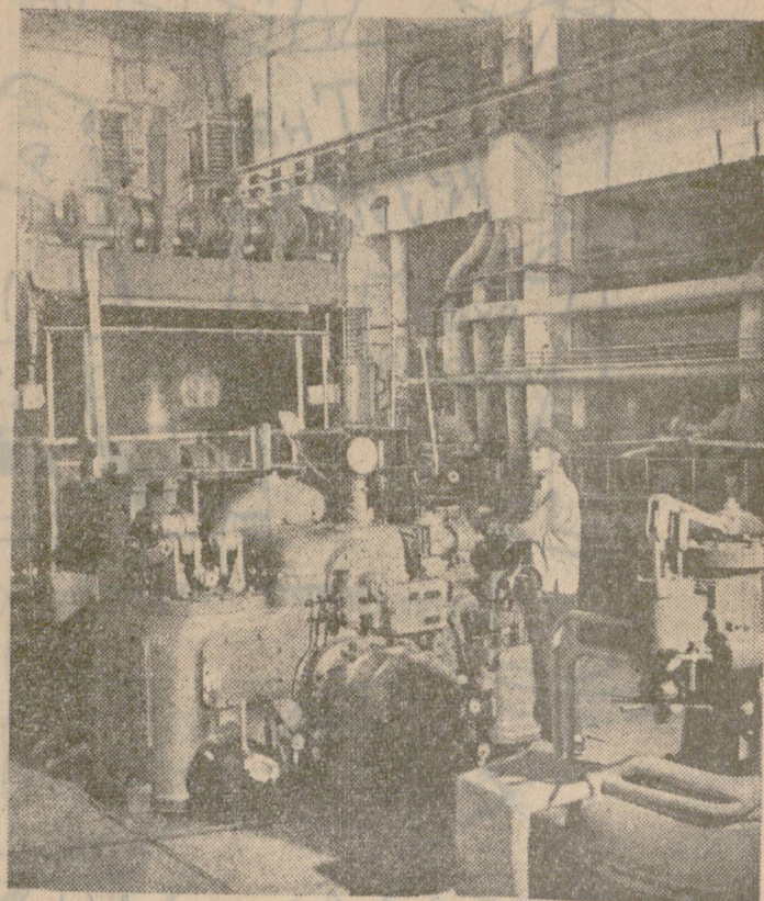
За гигантския икономически скок, който се извършва в Китайската народна република, бе необходима двигателна сила. И по всички краища като гъби изникнаха парни и водни електростанции. На снимката: В гр. Паоту неотворна влезе в експлоатация централа с начална мощност 25,000 киловата.
