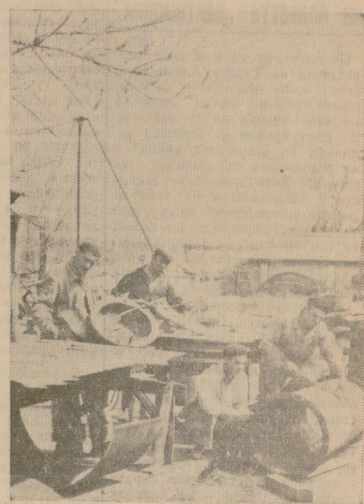
Бригадата на Н. Ганчев от ремонтната работилница при спиртната фабрика на ДЗЗ в Г. Оряховица монтира кондензатор за реконструиране на апарата „Рьом“ в „Борба“ и почистване на неговия капациет.
