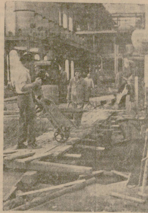
Работниците от Строителната организация в Горна Оряховица подготвят основите за монтиране на новите инсталации и машини в захарна фабрика на ДЗЗ Г. Оряховица.
