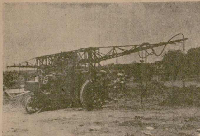
Нова, широкообхватна лозова пръкачка, производство на ДИП „Металургия“ — Г. Оряховица, пристигна наскоро в ТКЗС в с. Дъско. За два дни агрегатът вече е напъркал 600 декара лозови насаждения. Ново, голямо облекчение за кооператорите и за ускоряването на работата!
