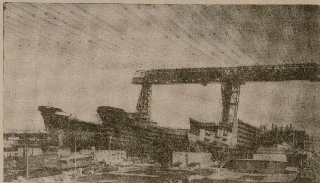
Най-големият в Европа, високият 65 метра кран в роцковската корабостроителница „Варноверфт“, с помощта на който едновременно се строят четири парахода.
