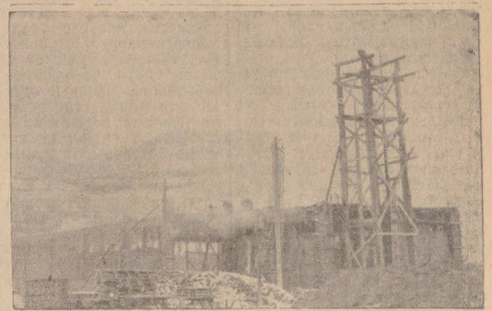
Въпреки студентите зимни дни строителството на новия завод за струно-бетонни траверси в гр. Свищов продължава. С всеки изминат ден все по-упорито се издигат корпусите на завода.
