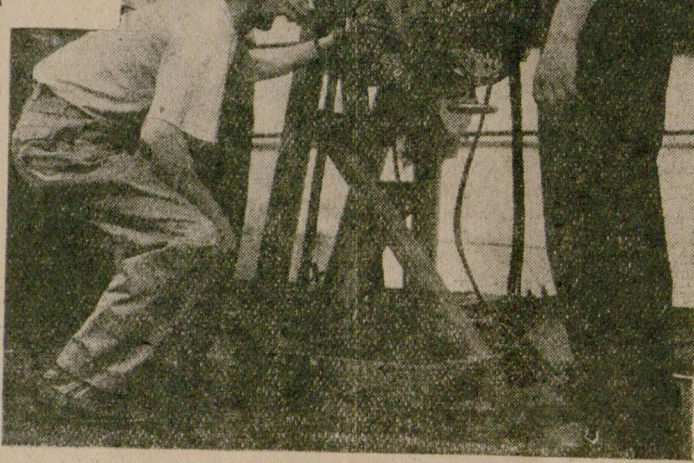
В павилиона „Машиностроене“. Посетители оглеждат тръбозаваръчен автомат, който позволява да се заваряват тръби с диаметър до 377 мм. Скоростта на заварката е до 100 м. в час. Снимка: А. Чернунов
