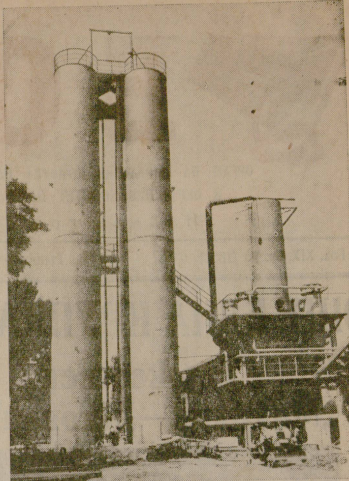
Новата инсталация в цеха за производството на въгледвукукс при Държавни захарни завод е едно голямо дело на социалистическата бригада за технически прогрес с ръководител инж. Байчев. Снимка Н. Качаков
