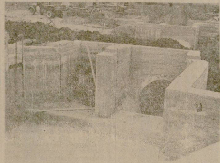
Предсрочно бе завършен един от най-трудните обекти по Десния главен напоителен канал от Росишката напоителна система, джокера под река Негованка край с. Русала.
