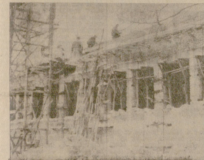
Строителната бригада на Крум Недялков въпреки големия студ не спира работата си по строежа на сградата за фура в с. Камен. НА СНИМКАТА: Бригадата довършва покривната конструкция.
