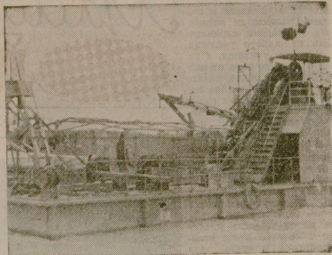
Така изглежда дълбачната „Алено“ от Българския драгажен флот.
