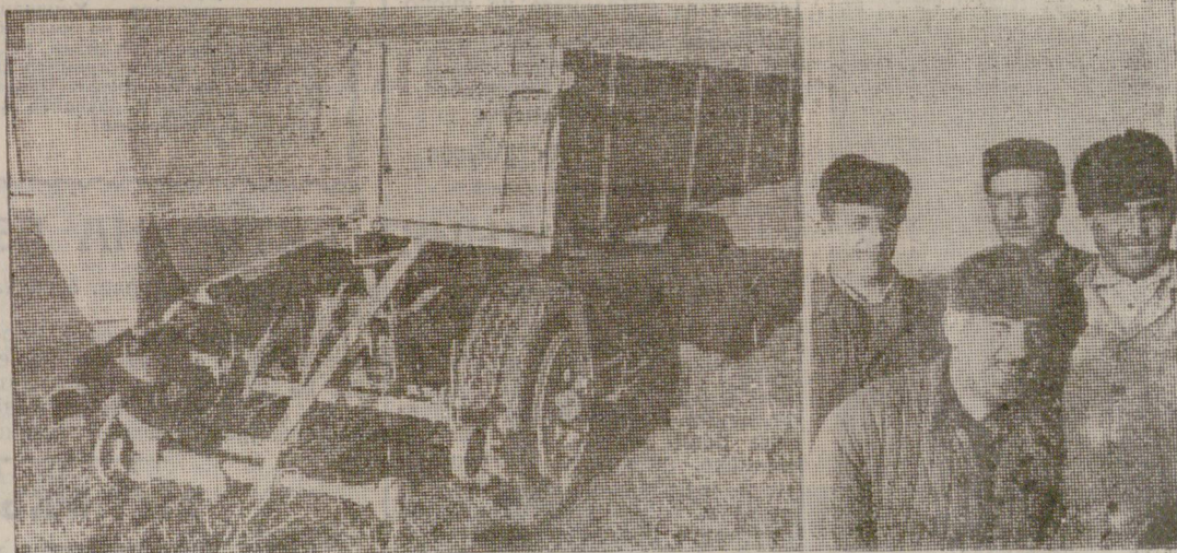
Механизаторите Никола Шопов, Стефан Върбанов, Йордан Кенчев и Иван Райков от с. Стрелец изработиха с подготвени материали центробежни тороразпръсвачка, която прикача на ремарке. С нея те могат да наторяват дневно до 800 декара посеви.
