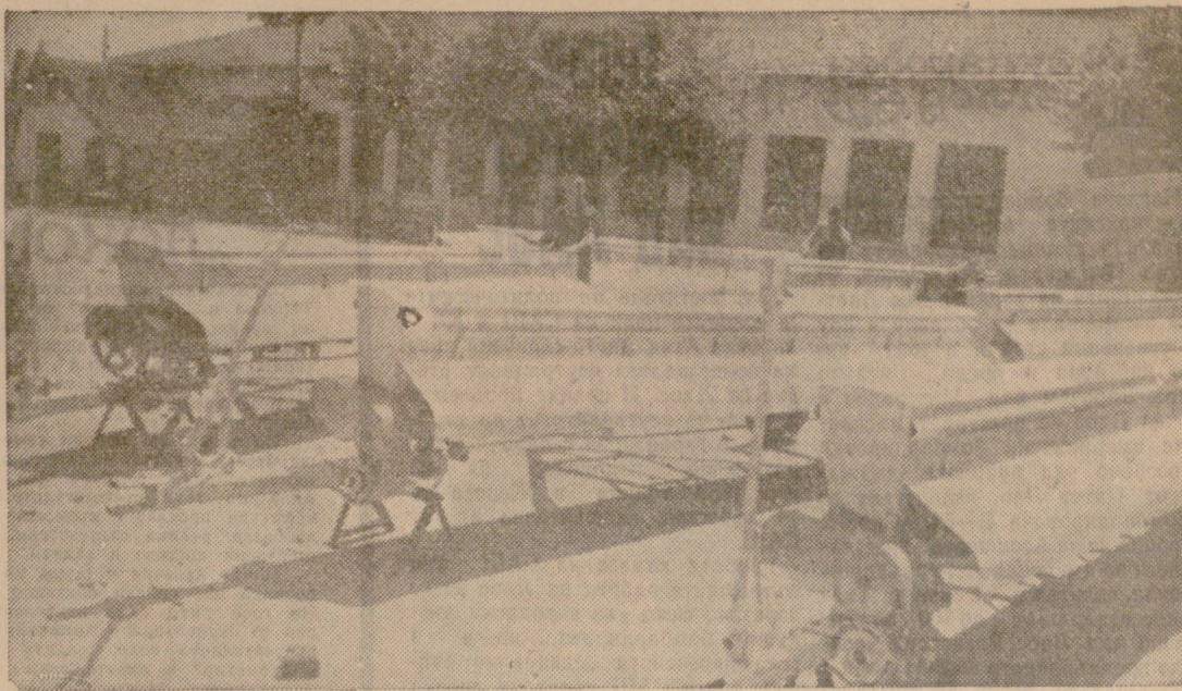
В ДМЗ „Първи май“ — Полски Тръмбеш от началото на второто шестмесечие започна серийно производство на широкообхватни тороразпръсвачки „ТТ-5“ с производителност от 14 до 35 декара на час и „ТРСШ-4“ с производителност от 12 до 28 декара на час. До края на годината ще се произведат общо 370 тороразпръсвачки.
