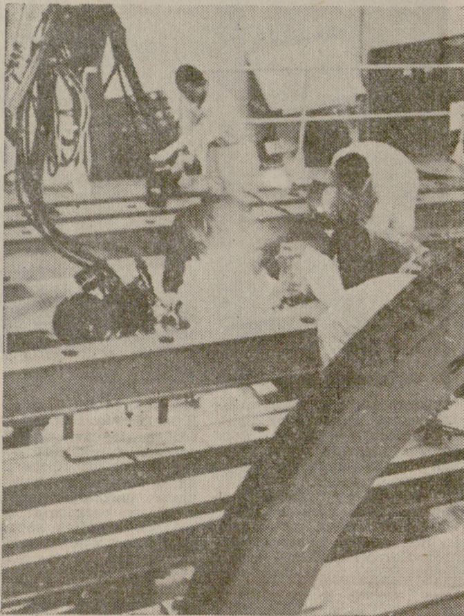
В заводите „Шкода“ в Пилзен е изработен резервоар за тежка вода, предназначен за ядрения реактор на първата чехословашка ядрена електроцентрала в Яслоуе-Букувице. ПРЕСФОТО — БТА
