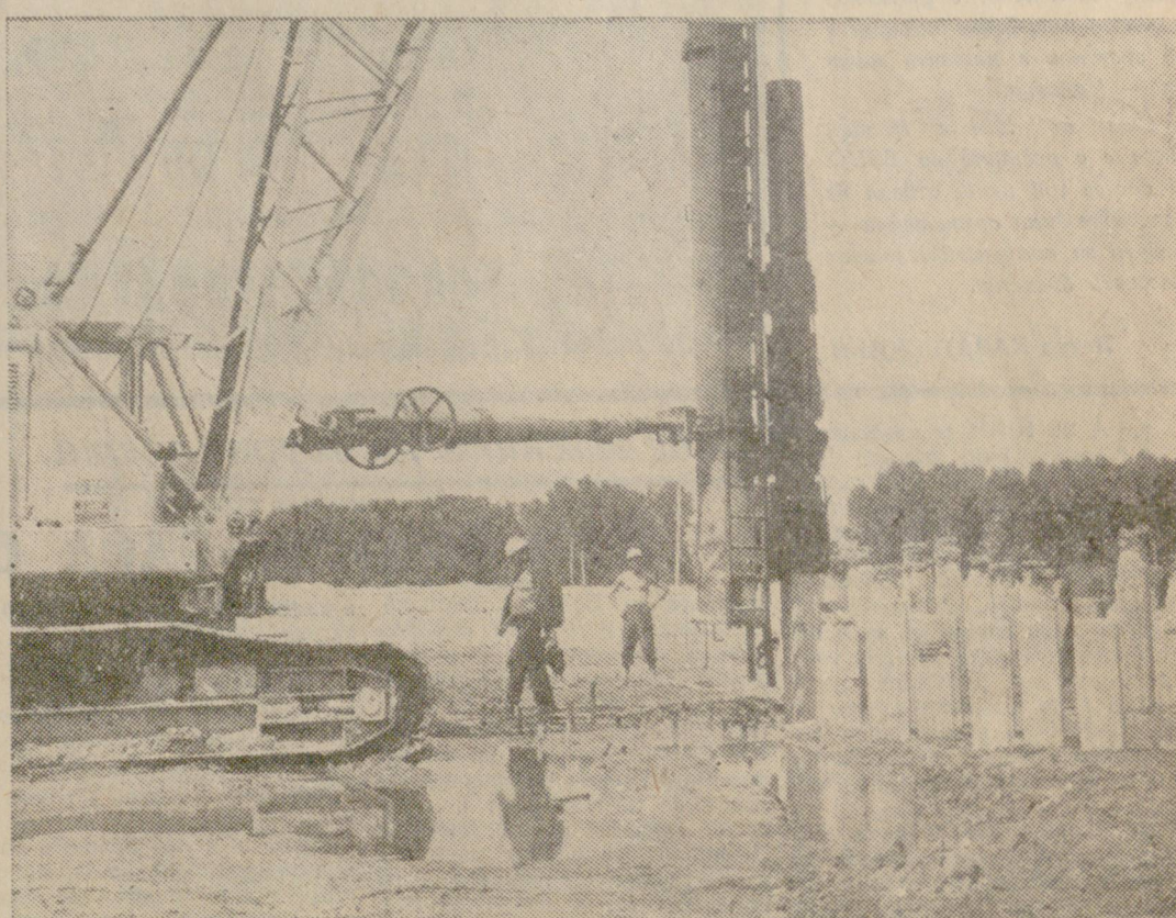
Трудна и отговорна е работата на звеното ръководено от Йон Иванов по набиването на пилони за ТЕЦ-а на Химическия комбинат в Свищов. Със стройната сонетка хората от звеното набиват за смяна по 10—12 пилони.
