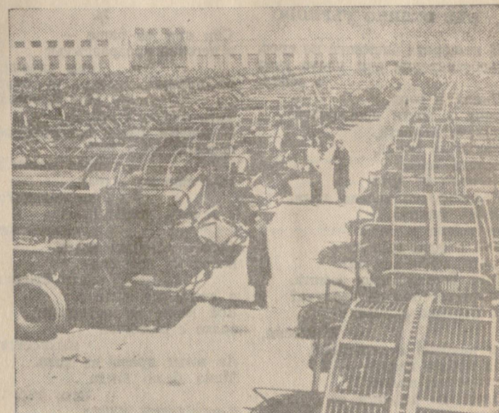
СССР. Рязанският завод за комбайни произвежда всеки месец повече от 500 комбайни за прибиране на картофи. Колективът на завода се готви сега за серийното производство на нов, по-съвършен комбайн за събиране на картофи ККУ-2 — „Дружба“.
