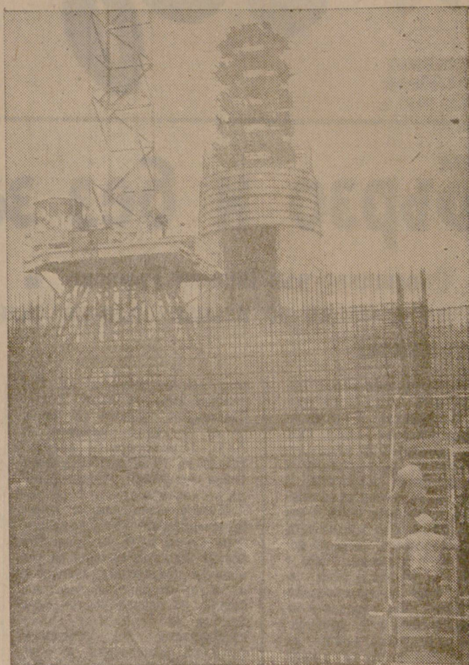
Напредва строежът на Атомната електроцентрала край гр. Кослодуй. Изграждат се съоръженията на втория реактор.
