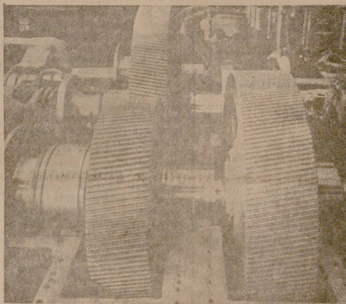
Работниците от заводите „Шкода“ в Пилзен, Западна Чехия са завършили третата трансмисия, предназначена за съветски риболовни кораби. На сн: бригада с ръководител Йозеф Хнат извършва монтажа на гигантската 73-тонна трансмисия.
