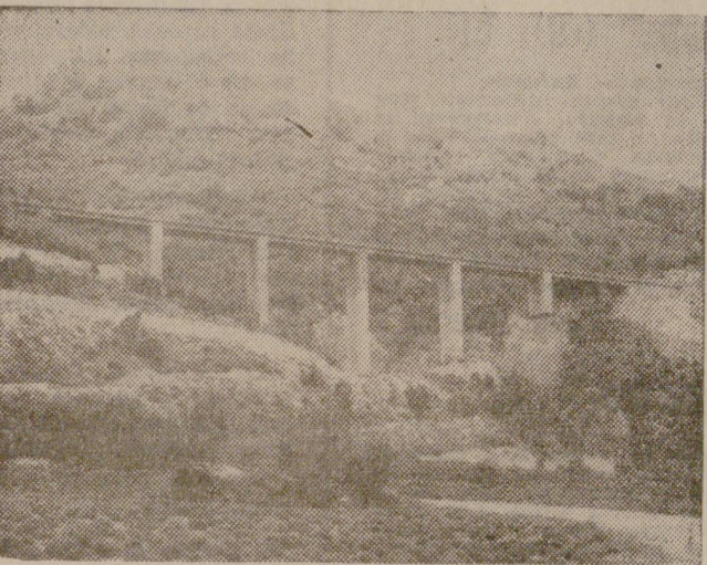
Наскорно влезе в експлоатация участъкът от пътята на гистрала София — Бургас край гр. Кансура. Тук са построени няколко големи моста по проект на инж. Лало Райков. На снимката: един от мостовете наречени „тип Камертон“.
