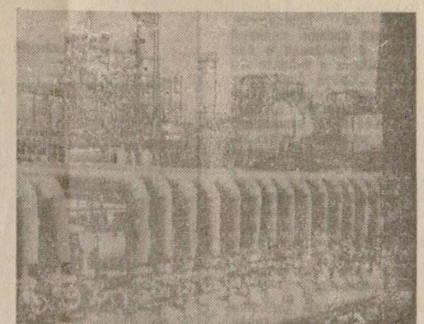
ГДР. На 9 юни 1972 година в цистерните на нефтохимическия комбинат в Швет, окръг Франкфурт на Одер протече 50-милионният светски суров нефт. На сн.: Изглед от нефтохимическия комбинат в Швет.
