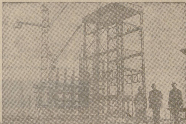
Първият пуск на парната турбина при ТЕЦ „Бобов дол“ трябва да бъде на 1 април 1973 г., вторият пуск през декември 1973 г., и третият — през юни 1974 г. Заедно с четвъртата турбина ТЕЦ „Бобов дол“ ще има мощност 840 мегавата.
