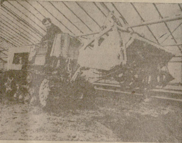
Научни сътрудници от Москва създадоха машина за основна и предпосевна обработка на почвата в парниците при отглеждане на зеленчуци, цветя и билки
