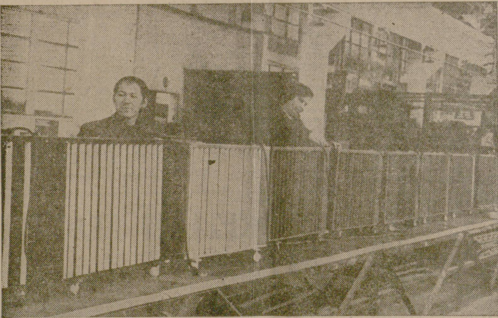
На конвейера за последен монтаж в Завода за радиатори — Стражица са новите електрически радиатори „Вега-3“ и „Вега-5“.
