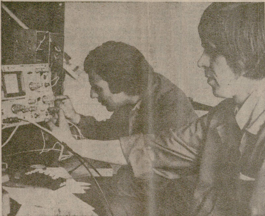
С всяка измината година расте броят на разработките—дело на членовете на клуба за ТНТМ към СХК „Свилюза“ — Свищов. Голям интерес предизвикват електронният брояч на импулси и характеристиката за полупроводников елемент, изработени от инж. Лилко Антонов и майстор Снимка Оник МИНАСЯН
